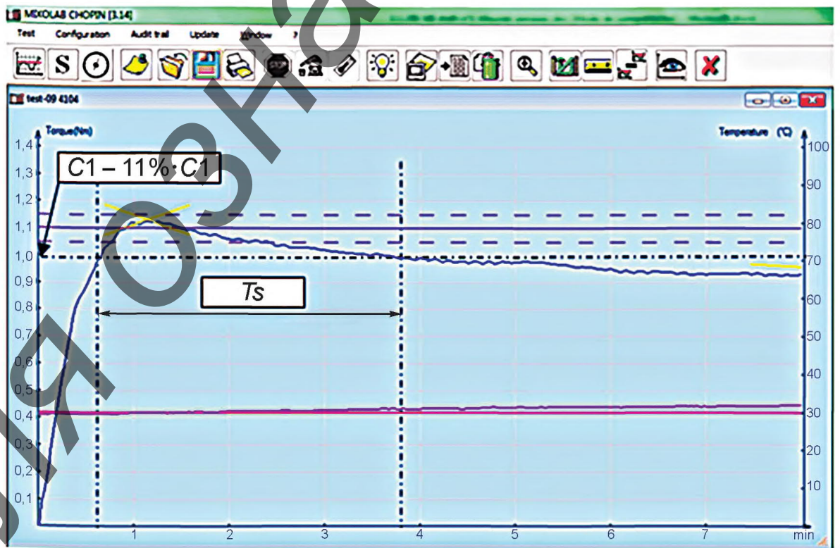
Рисунок А.2 — Расположение значений времени T_1 и температуры теста на кривой «Миксолаба»
